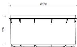
Rysunek 2: Nadbudowa D400 H200 AQ (kod wyrobu 2484 ).
