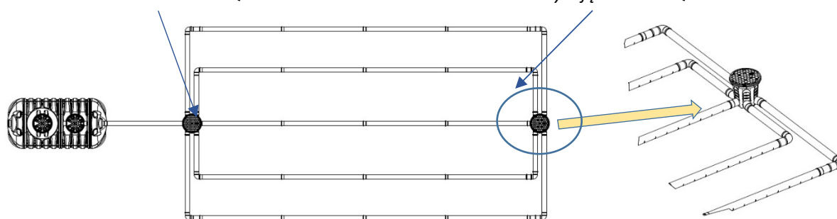
Rysunek 1: Studzienka zamykająca D400 AQZ – umiejscowienie w złożu rozsączającym
