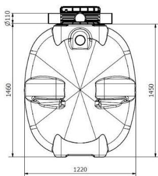
Rysunek 4: Zbiornik na wodę deszczową 3000 AB i 4000 AB – wymiary charakterystyczne
