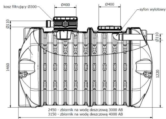
Rysunek 4: Zbiornik na wodę deszczową 3000 AB i 4000 AB – wymiary charakterystyczne
