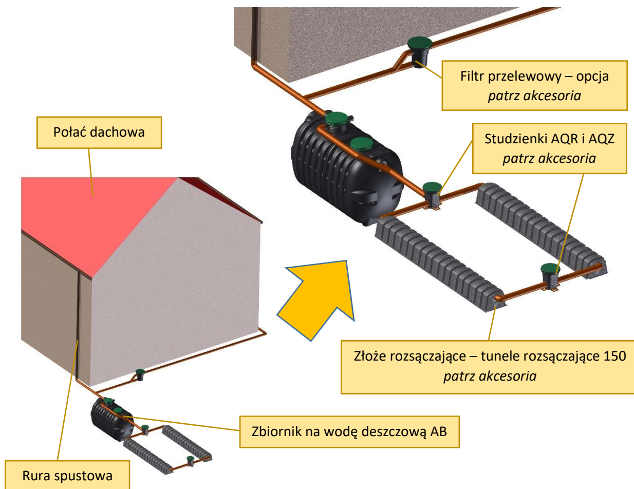
Rysunek 5: Instalacja zbiornika na wodę deszczową AB wraz ze złożem rozsączającym oraz opcjonalnym filtrem przelewowym przy domu jednorodzinnym o powierzchni dachu większej niż 150m 2
