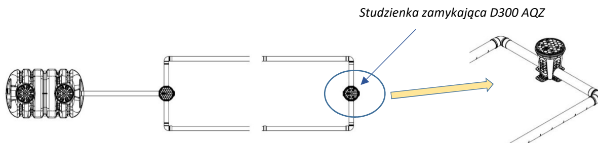
Rysunek 9: Studzienka zamykająca D300 AQZ – umiejscowienie w złożu rozsączającym
