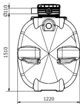
Rysunek 3: Zbiornik na wodę deszczową 2000 AB – wymiary charakterystyczne
