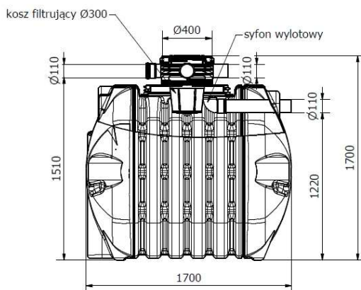
Rysunek 3: Zbiornik na wodę deszczową 2000 AB – wymiary charakterystyczne
