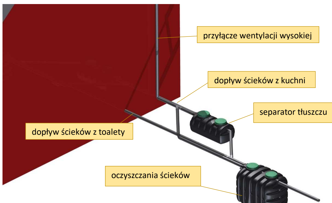
Rysunek 3: Instalacja separatora tłuszczu SL-SG przy domu jednorodzinym.
