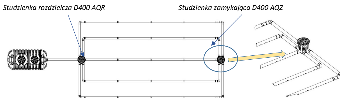
Rysunek 1: Studzienka zamykająca D400 AQZ – umiejscowienie w złożu rozsączającym
